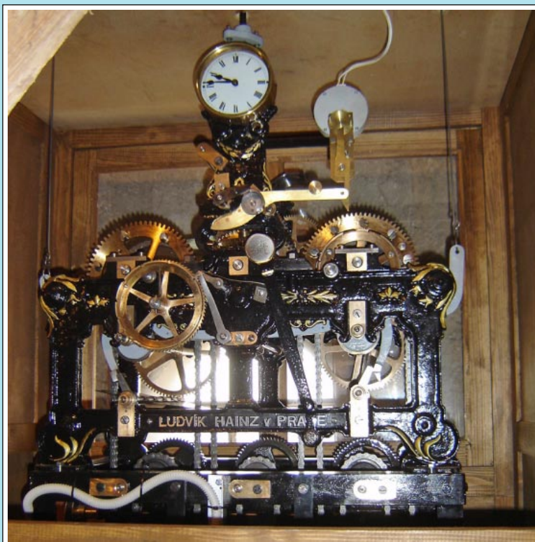
"Hodinový stroj po opravě a modernizaci"
