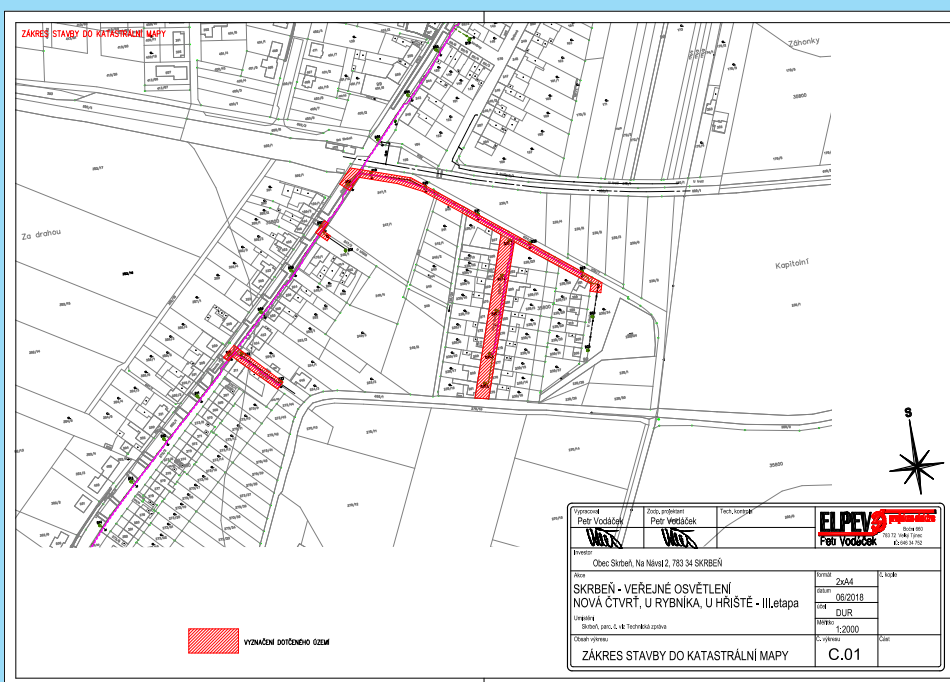
Projekt veřejného osvětlení v ulicích Nová čtvrť, U Rybníka a U Hřiště
